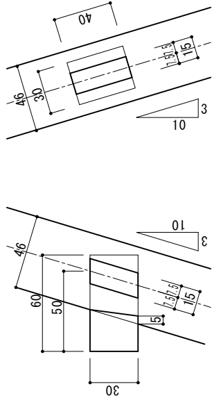
側面図による A.B.C.真詳細図
